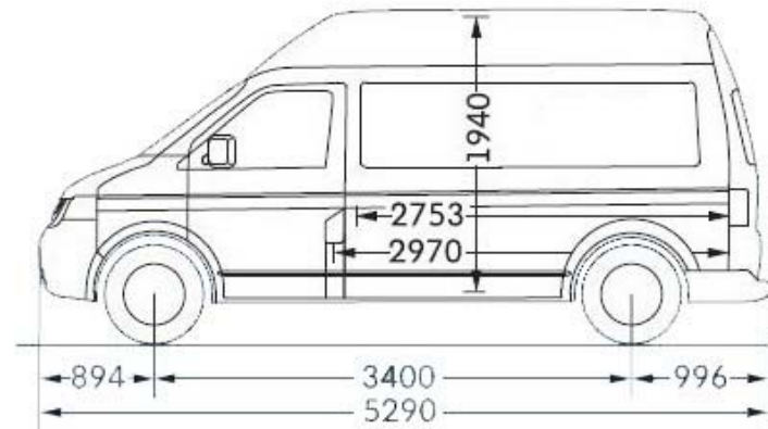
Lang Superhochdach
