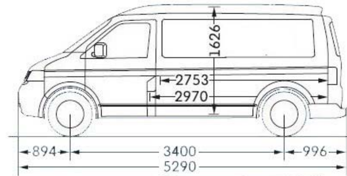
Lang Hochdach
